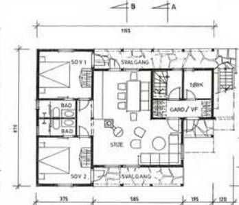
PLAN 1. ETASJE
