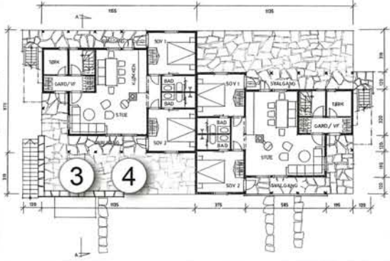
PLAN 1. ETASJE
